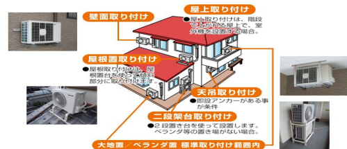
エアコン工事設置例
